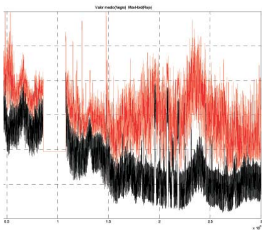
Gráficas 3. Medida Pico-Promedio y TFN de la medida AVC en banda B1
