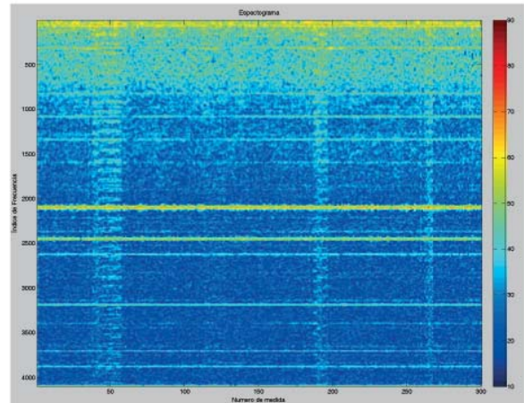
Gráficas 1 Medida Pico-Promedio y espectrograma de la medida de ruido en banda B1
