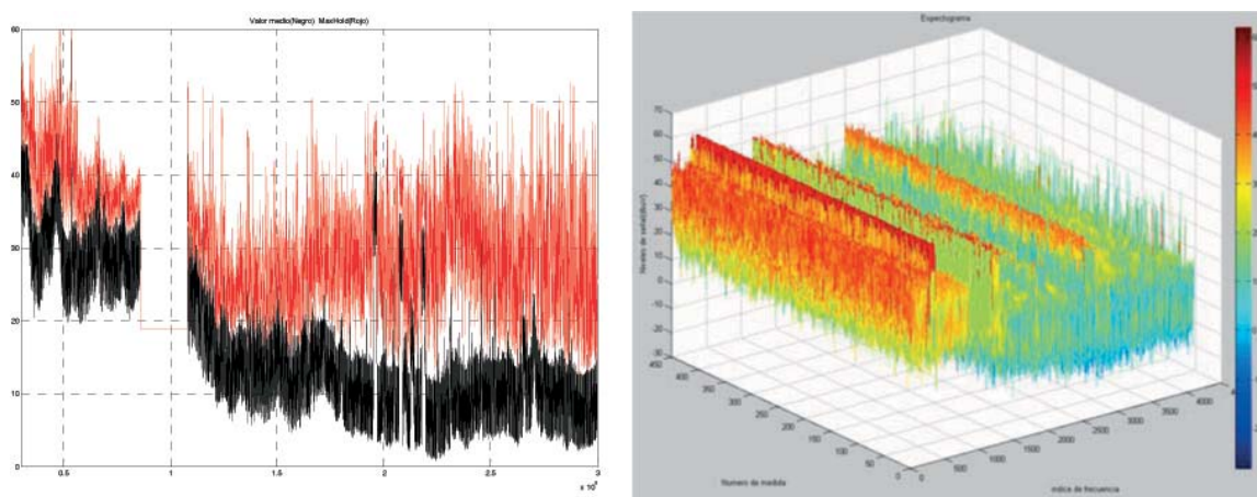
Gráficas 4. Medida Pico-Promedio y TFN de la medida AVC en banda
